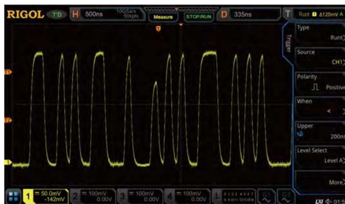
Запуск по импульсу нетипичной амплитуды поможет захватить нужный сигнал в последовательности импульсов.
